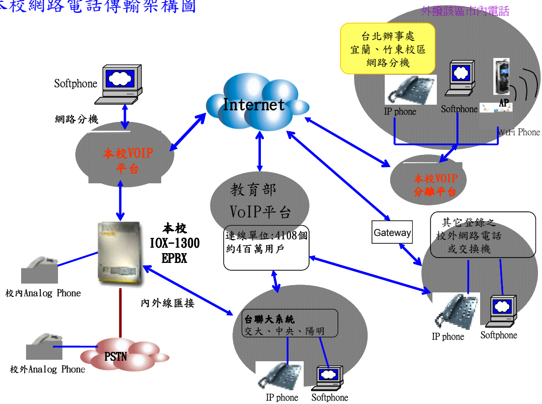
本校網路電話傳輸架構圖
